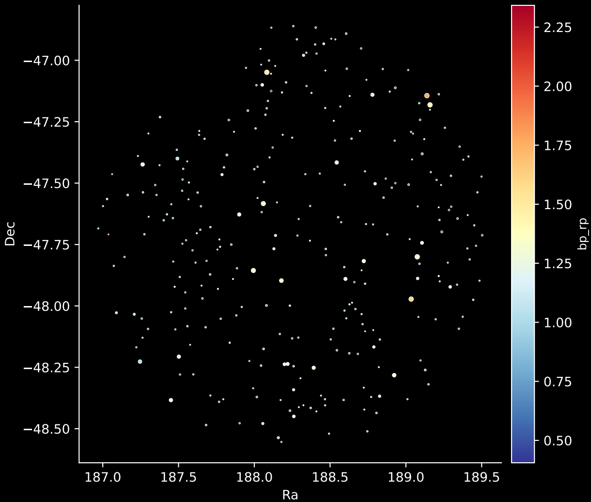
GALAH DR4 Field: [989] Stars: 290
