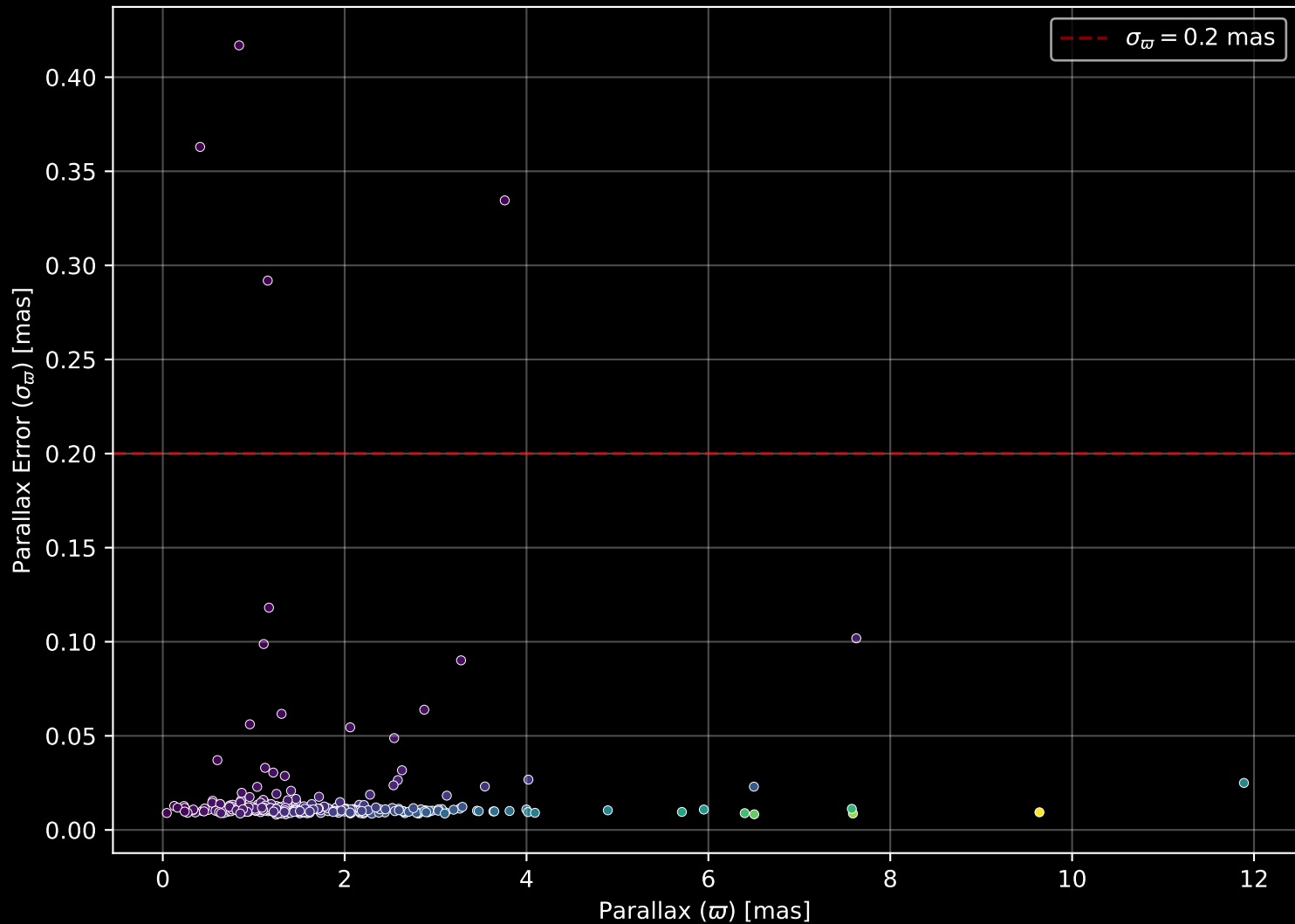
GALAH DR4 Field: [989] Parallax Quality (n= 290)
