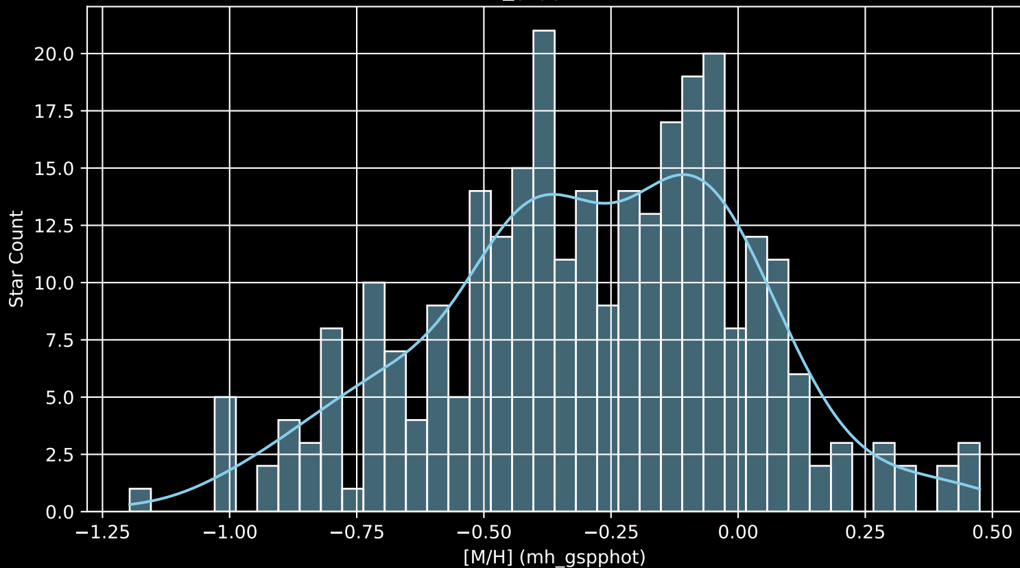
GALAH DR4 Field: [989] [M/H] (mh_gspphot) (n= 290)
