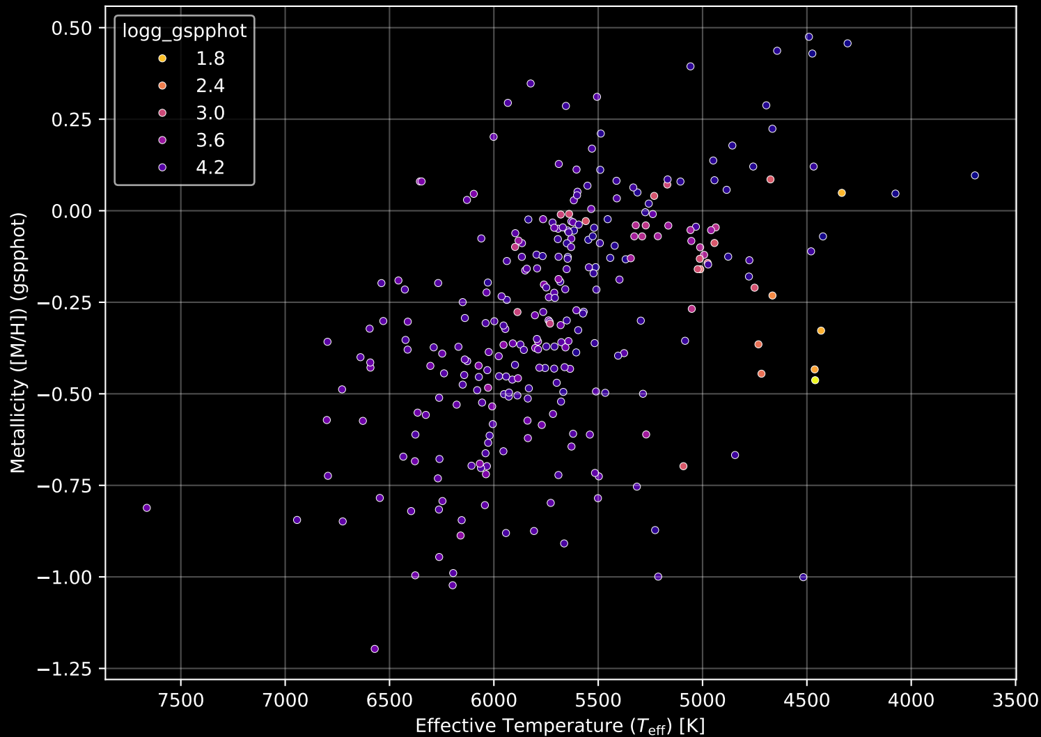
GALAH DR4 Field: [989] Stellar Population Parameters (n= 290)
